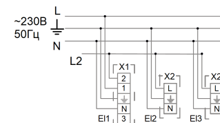
Схема подключения нескольких светильников
